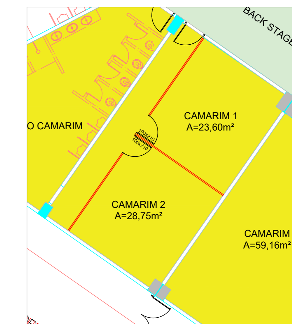
CAMARIM 01 E 02 - BACK STAGE esc. 1/100
