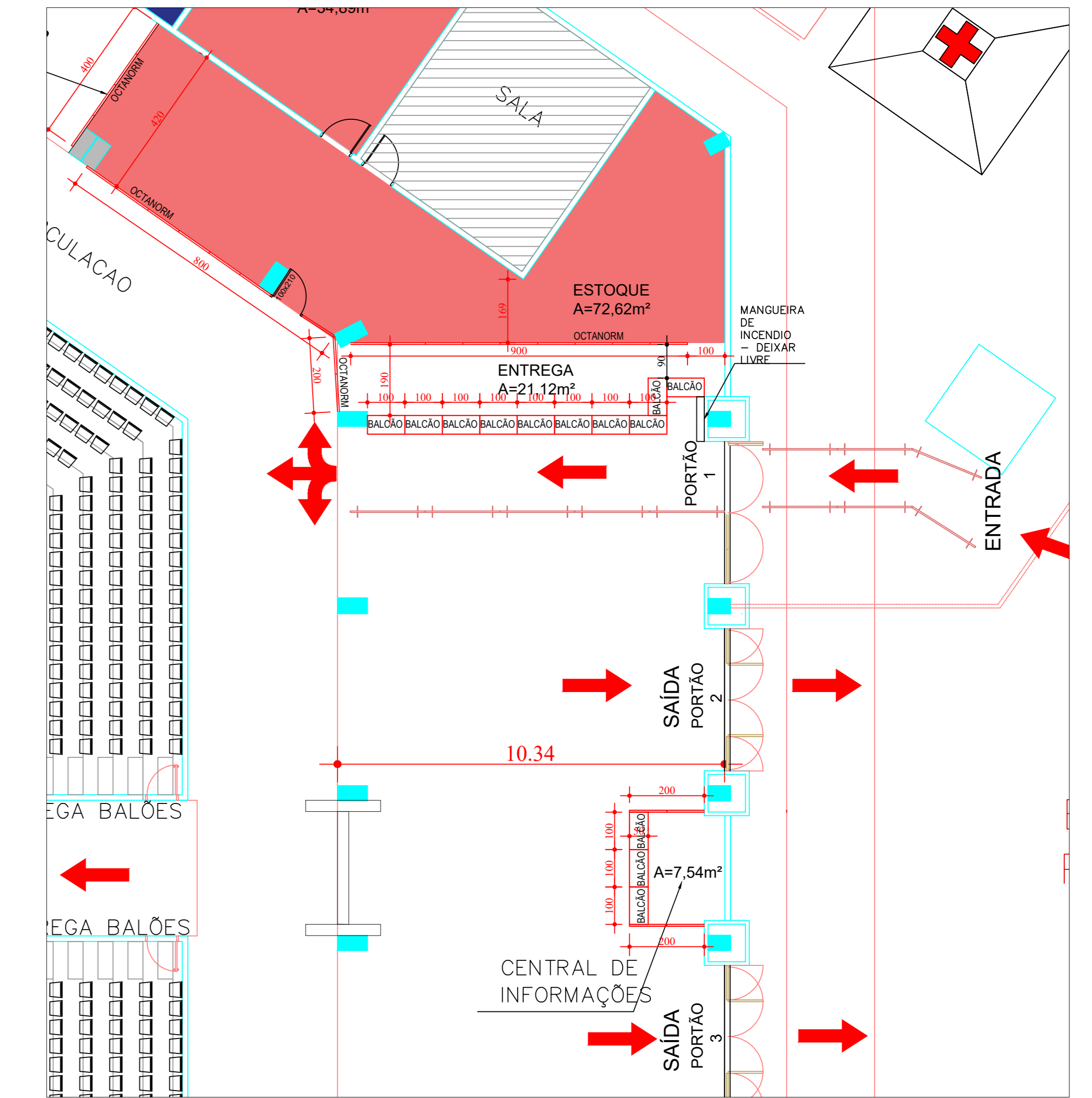
PORTÕES 01 E 02 - CADEIRAS esc. 1/100
