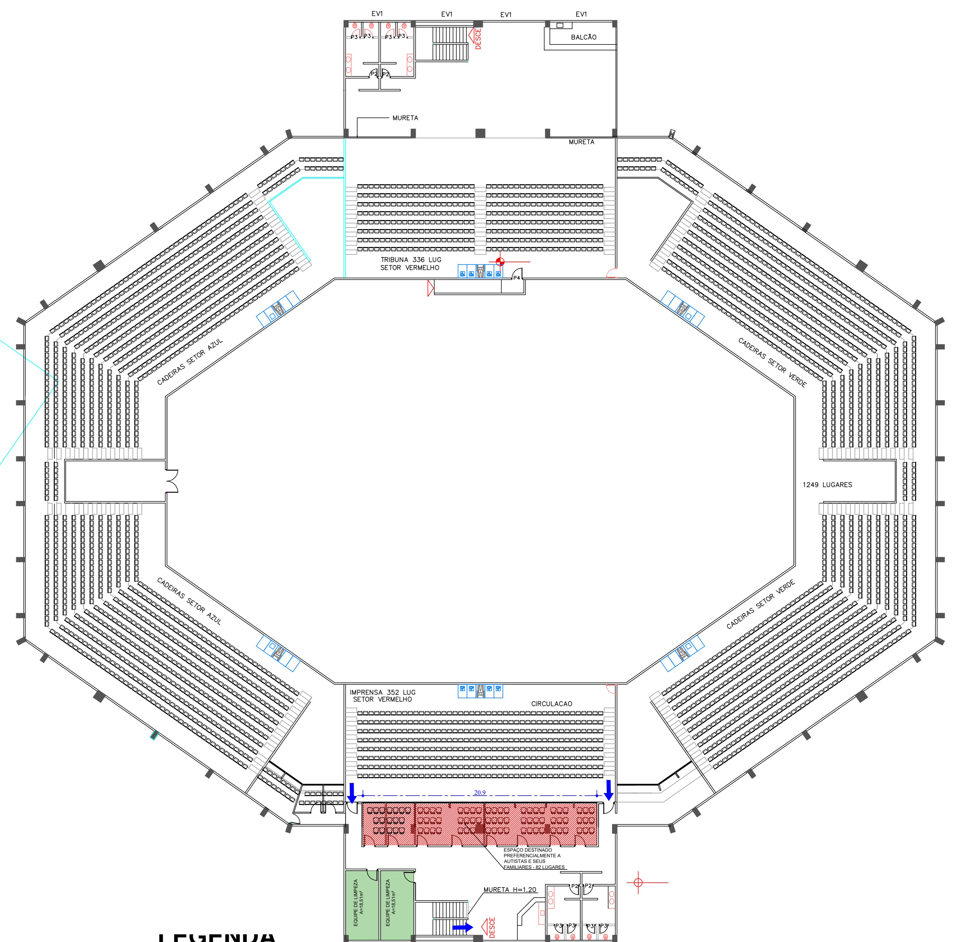
PLANTA NÍVEL TRIBUNA esc. 1/200
