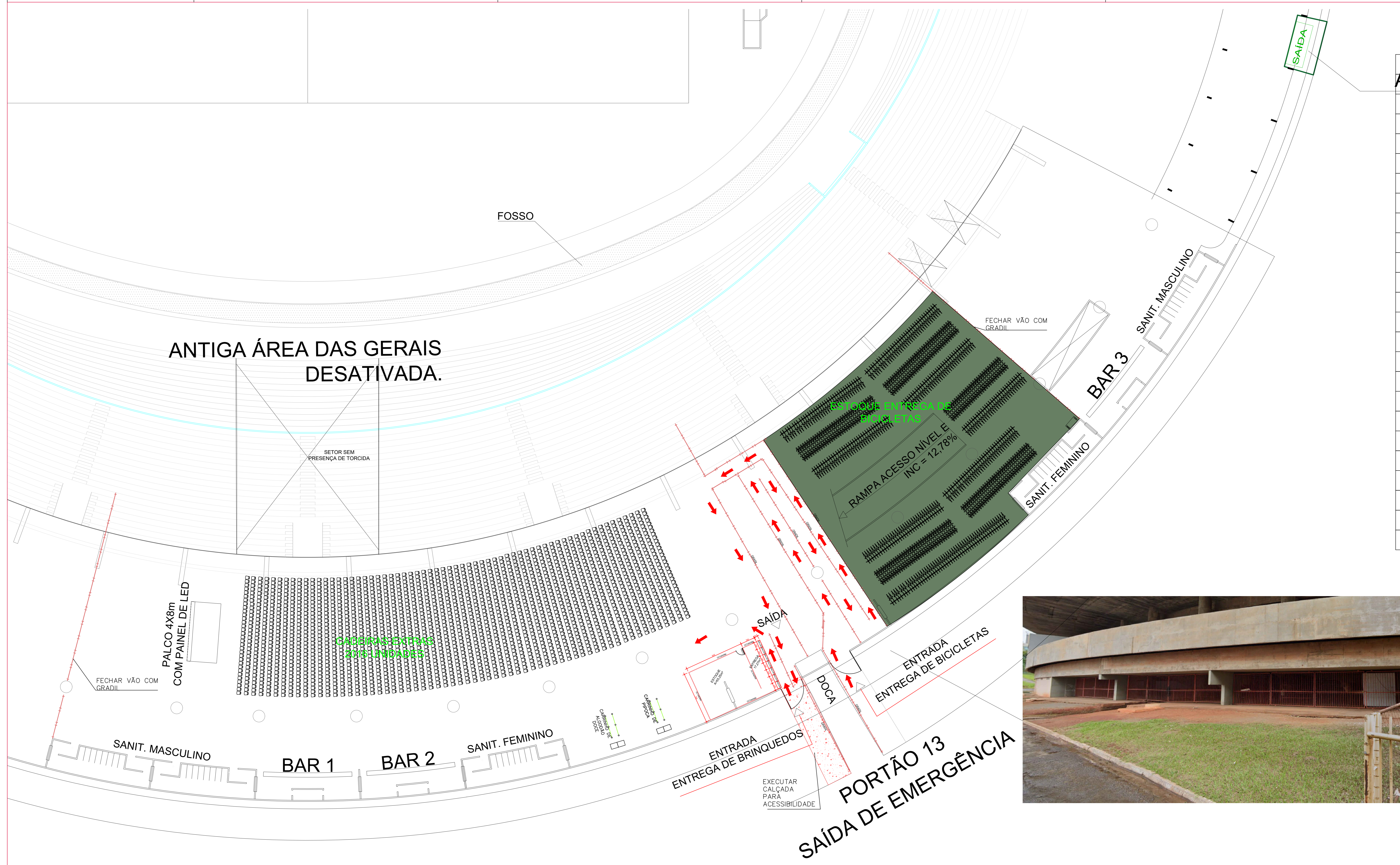
PLANTA ANEXO SERRA DOURADA esc. 1/200
