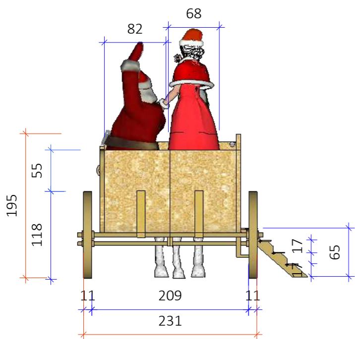
VISTA POSTERIOR Esc.: 1/50
