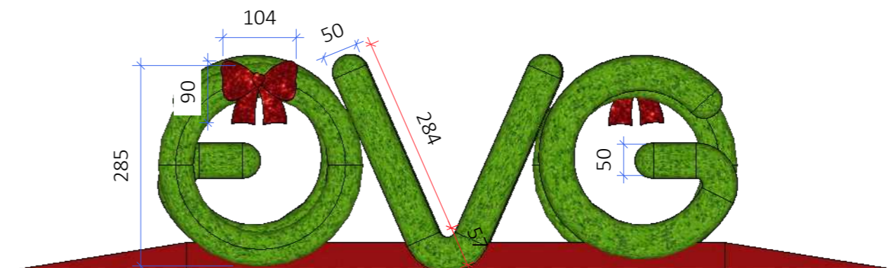
VISTA FRONTAL Esc.: 1/100
