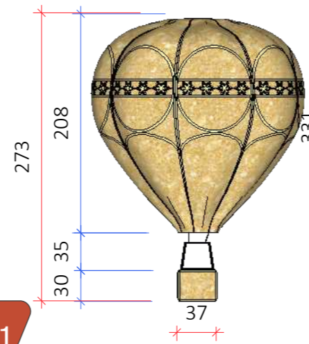
VISTA FRONTAL Esc.: 1/75
