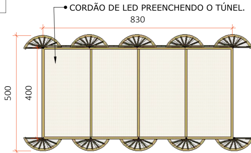
VISTA POSTERIOR Esc.: 1/50
