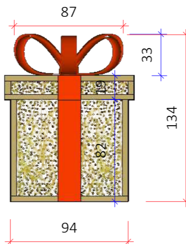
VISTA FRONTAL Esc.: 1/30
