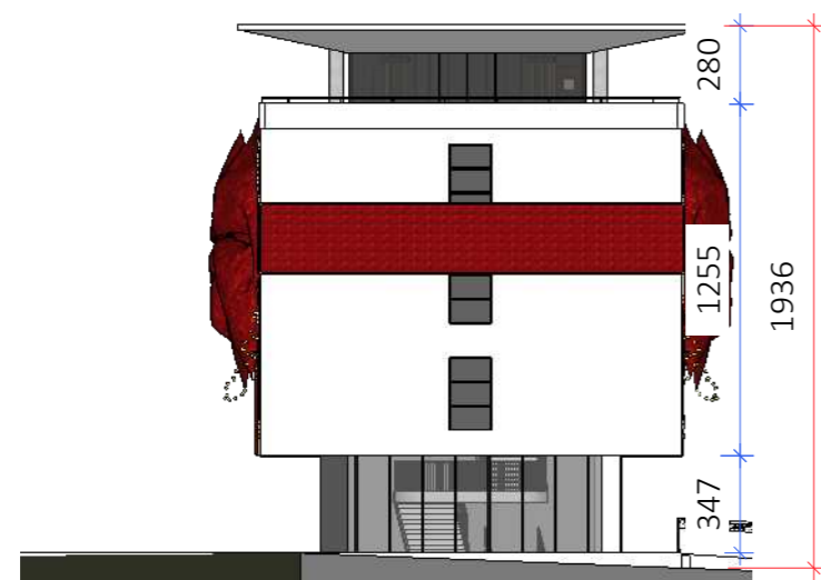
VISTA B- LATERAL DIREITA- BIBLIOTECA Esc.: 1/300
