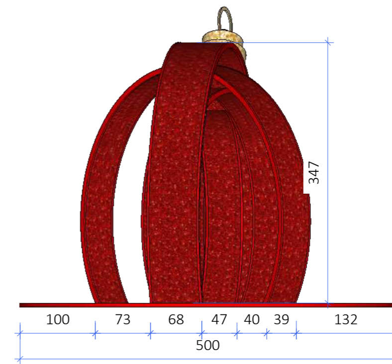
VISTA LATERAL Esc.: 1/50
