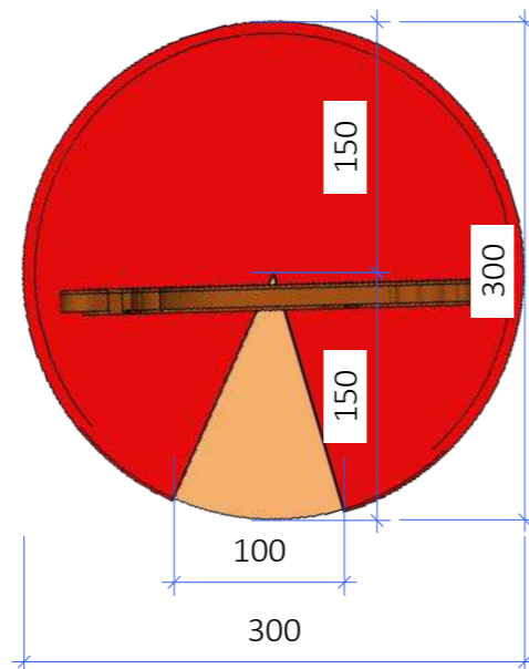
VISTA SUPERIOR Esc.: 1/50
