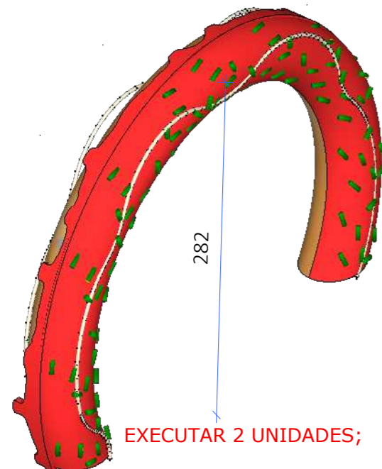
PERSPECTIVA Esc.: 1/30
