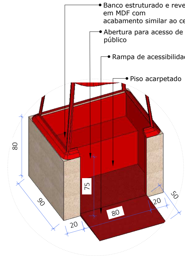
DETALHE- CESTO Esc.: 1/50
