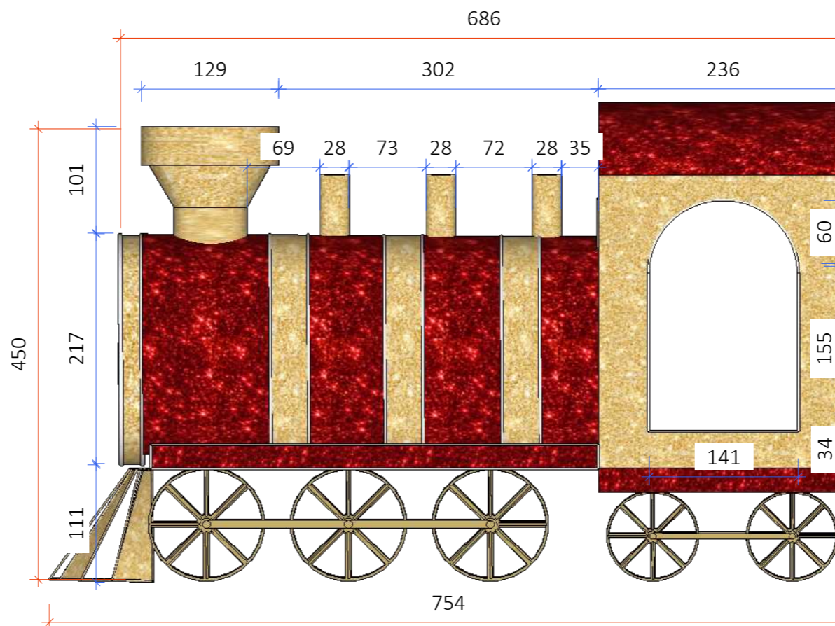
VISTA LATERAL Esc.: 1/50
