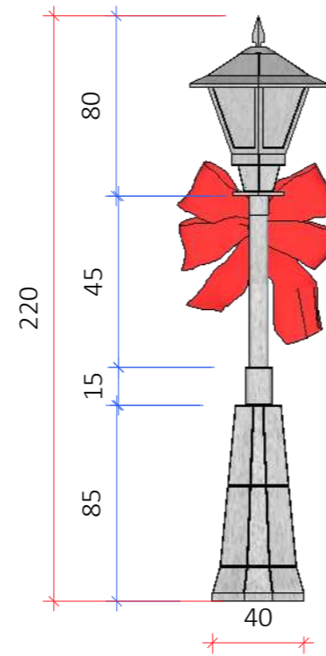
VISTA FRONTAL Esc.: 1/30
