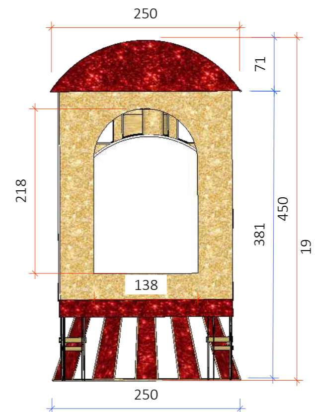
VISTA POSTERIOR Esc.: 1/50
