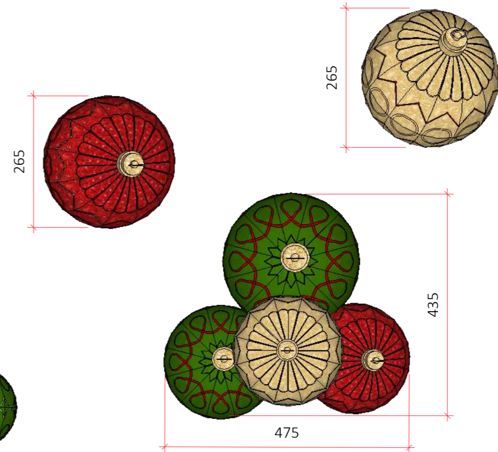
VISTA SUPERIOR Esc.: 1/75
