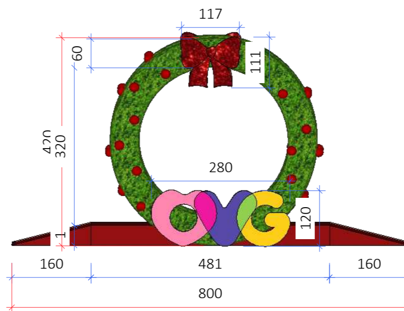
VISTA FRONTAL Esc.: 1/100
