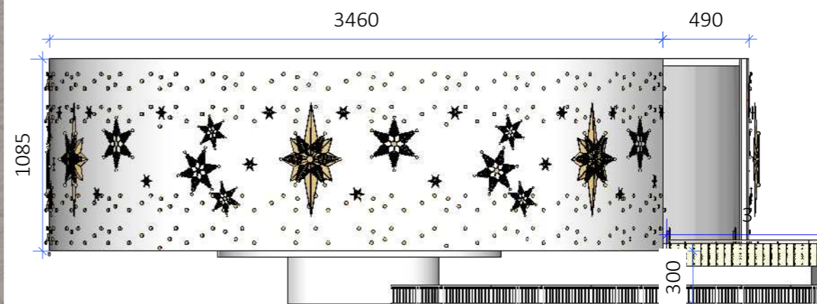
VISTA D - FACHADA POSTERIOR- MUSEU Esc.: 1/300
