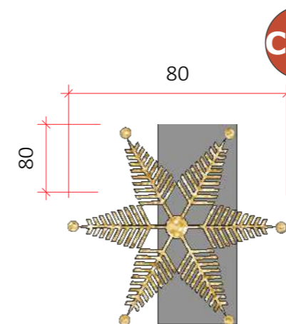
VISTA FRONTAL - ESTRELA P Esc.: 1/15
