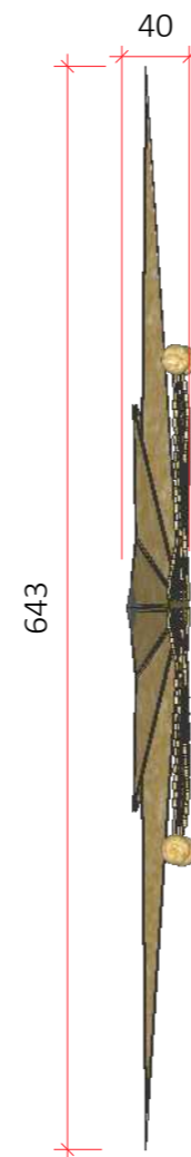
VISTA LATERAL - ESTRELA G Esc.: 1/50
