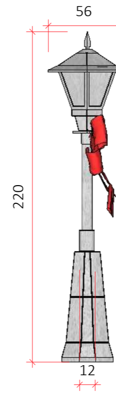
LATERAL Esc.: 1/30
