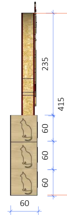
VISTA LATERAL Esc.: 1/50
