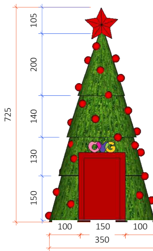
VISTA LATERAL Esc.: 1/75
