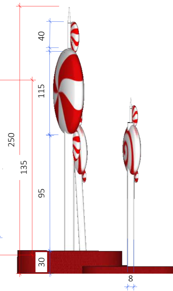
VISTA LATERAL Esc.: 1/30
