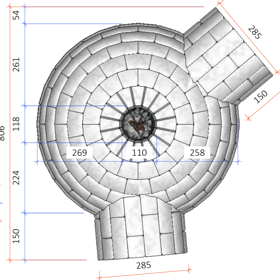
VISTA SUPERIOR Esc.: 1/75
