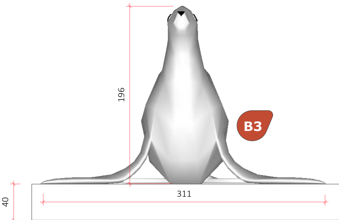
VISTA FRONTAL - MORSA Esc.: 1/25
