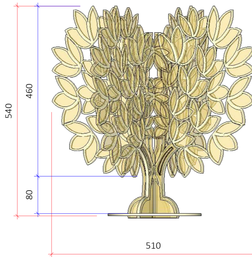
VISTA FRONTAL Esc.: 1/50
