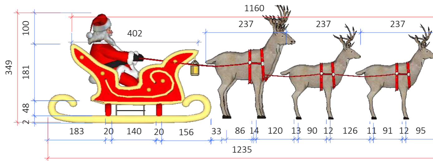
VISTA LATERAL Esc.: 1/75
