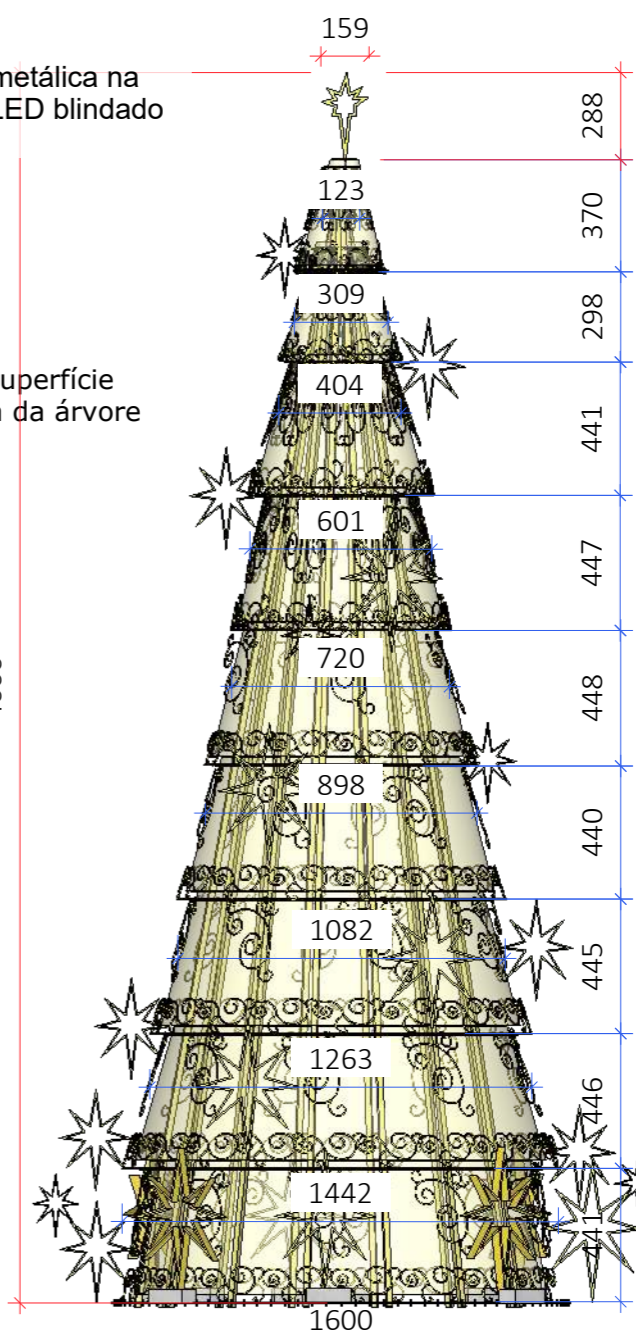
VISTA FRONTAL Esc.: 1/250
