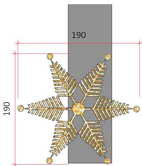
VISTA FRONTAL - ESTRELA M Esc.: 1/15
