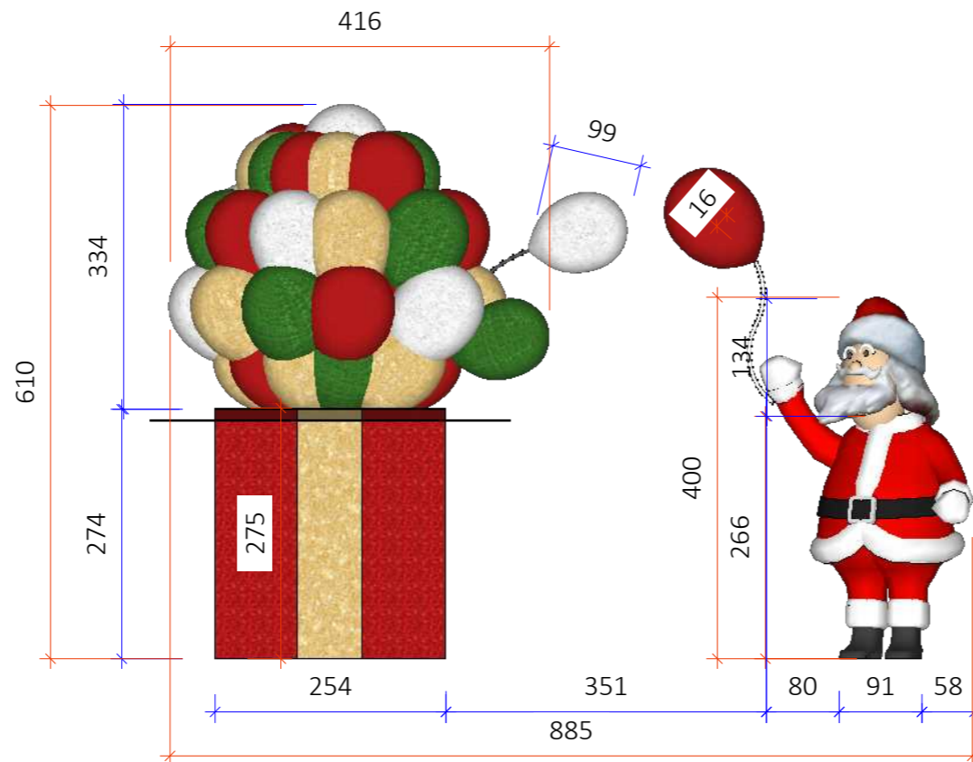
VISTA FRONTAL Esc.: 1/75
